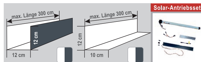
Abb.: Korrosionsbeständige U- oder L-Profile aus Aluminium als Sicht- und Spritzwasserschutz und zur Befestigung eines Solarpanels beim Einsatz unseres Solar-Antriebssets.
